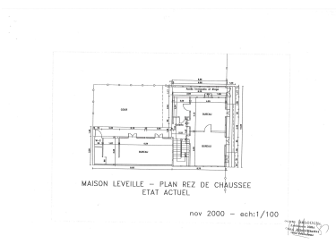
Plan du rez-de-chauss e, Sonia Delouche architecte, 2000. Phot. Sonia Delouche IVR03_202697300203NUCA
