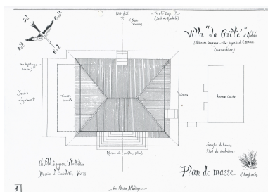
Plan de masse dressé par Ch. Vidal, février 1993
