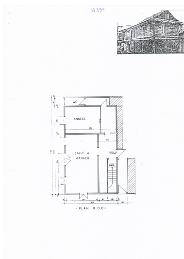
Plan du rez-de-chaussée, relevé conseil général, 1995 IVR03_202697300199NUCA
