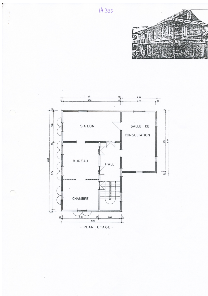
Plan de l'étage, relevé conseil général, 1995
