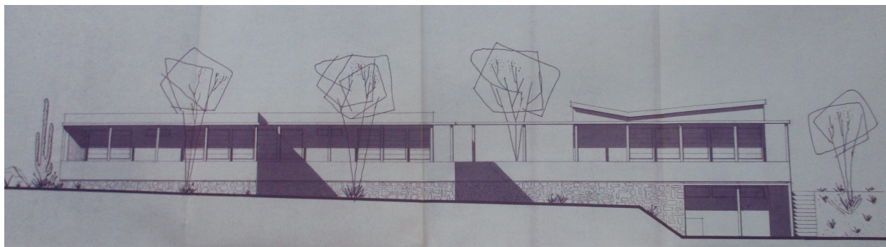
Extrait du plan déposé en 1965, façade sud vers la mer
