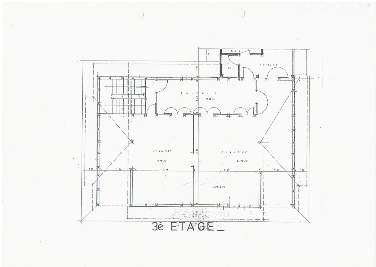
Plan du troisième étage sous comble, dossier de restauration CRMH, vers 1991
