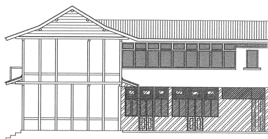
MAISON LEVEILLE – PIGNON DROIT
